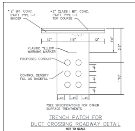
conduit trench detail
